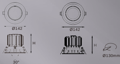
FS5070-30
